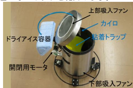
蚊のオートサンプリングマシン
