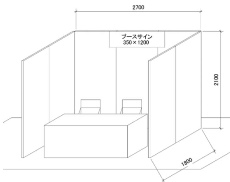
図 1: ブースレイアウト（テーブル 1 台 (W1800×D600×H700)・イス 2 脚）
